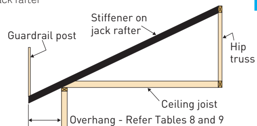
c) Jack rafter
