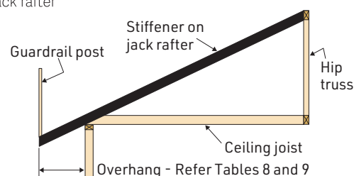
c) Jack rafter
